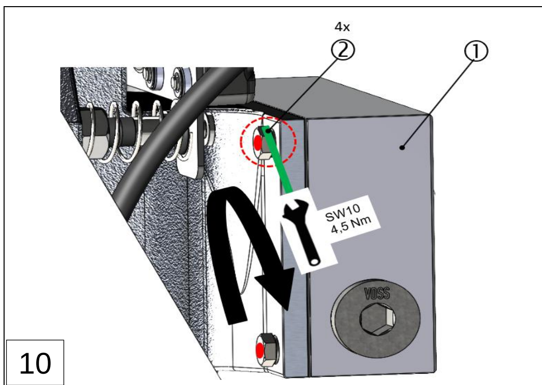
1: Anschlusskasten
