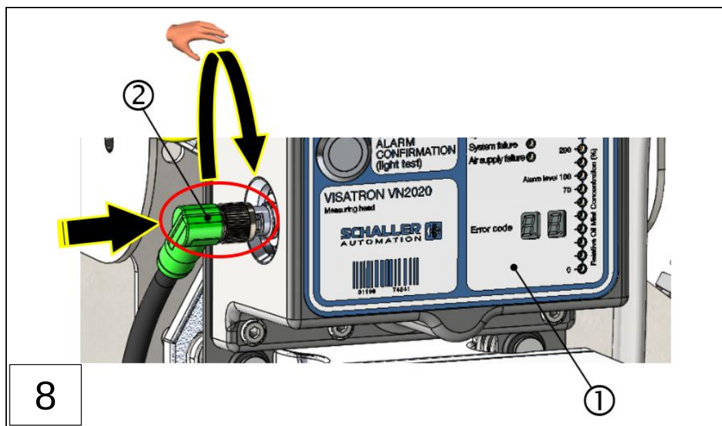
1: Messaufsatz, VN2020
