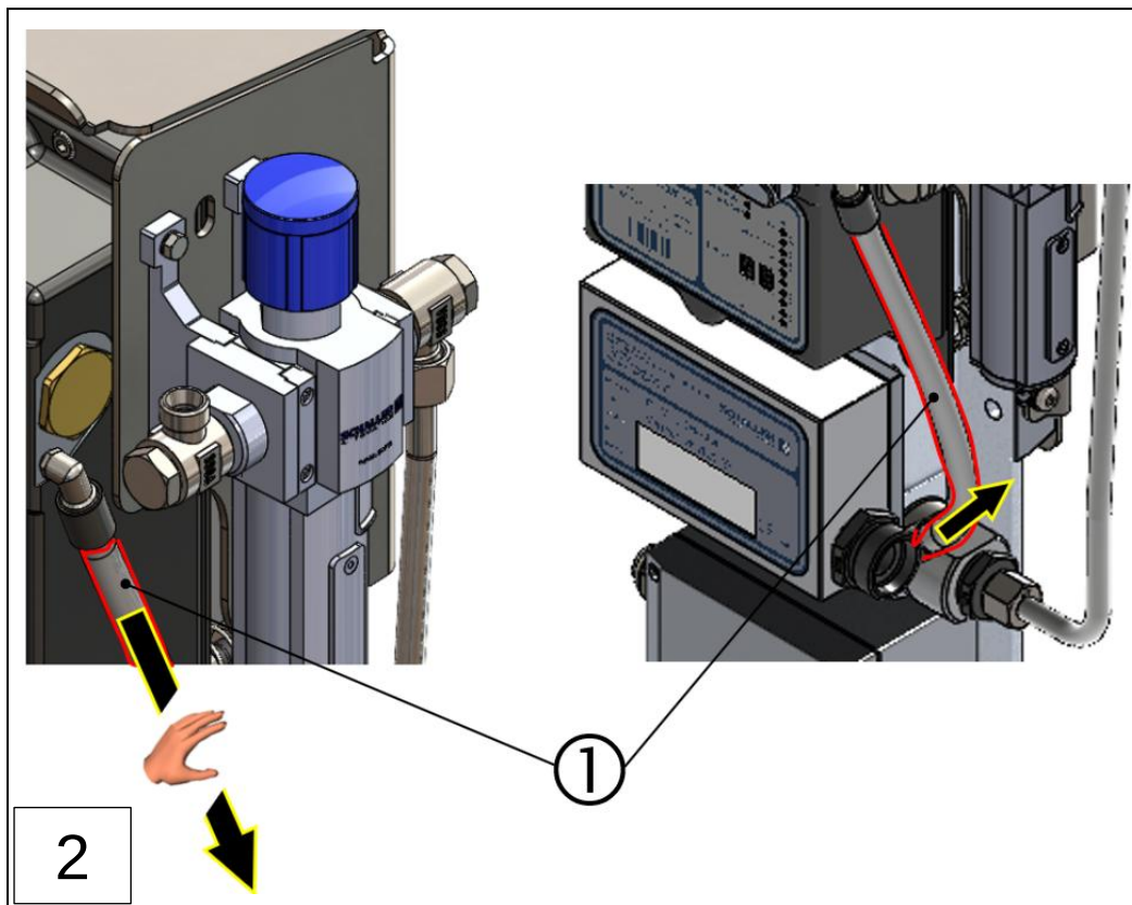
1: Verbindungsschlauch (alt)
