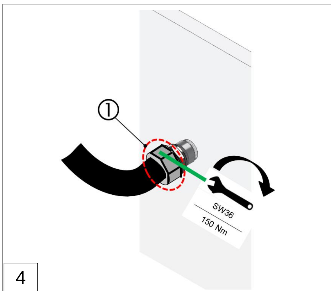
Abb.: 36 : Montage der Rückführungsleitung, VN2020 (Schritte 1-4)
