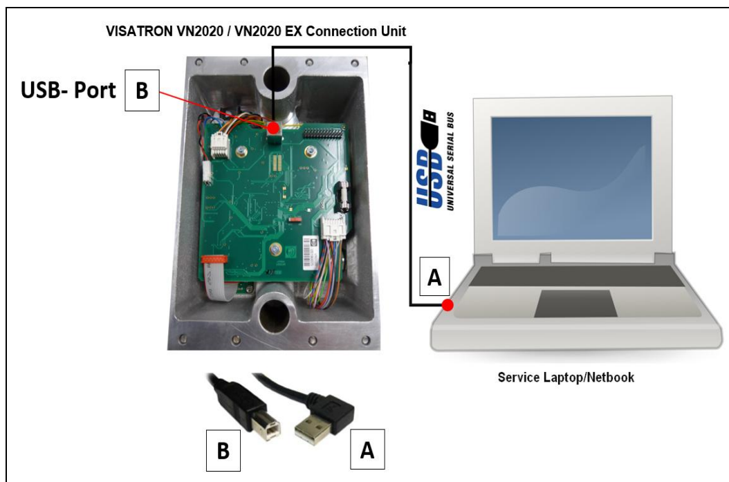
Abb.: 67 : Herstellen der USB- Verbindung zwischen Messaufsatz VN2020 und Service- PC
