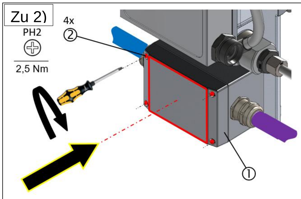
Abb.: 89 : Klemmenkasten austauschen, VN200 (Montageschritte 1- 8)
