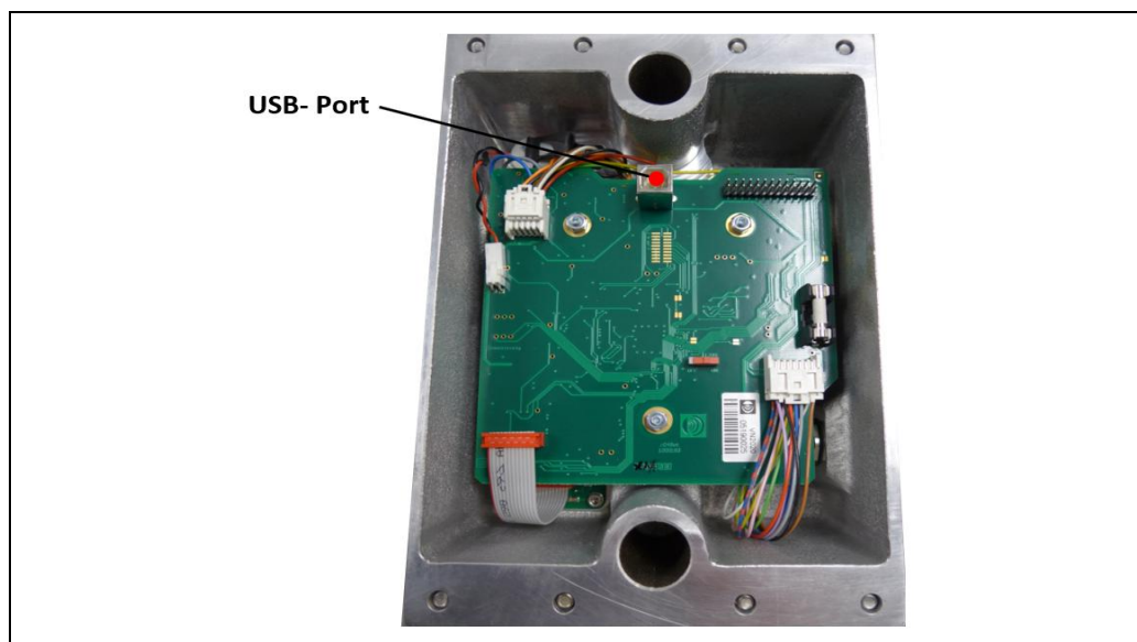
Abb.: 65 :Messaufsatz VN2020, Ansicht Rückseite, USB- Port
