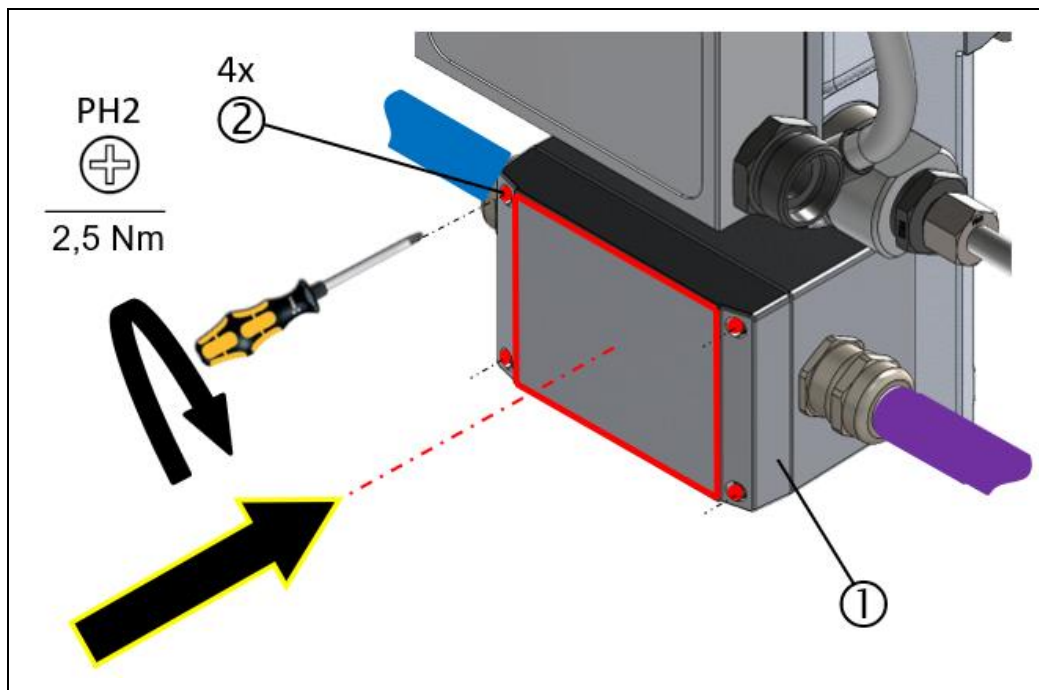
Abb.: 53 :Verschließen des Klemmenkastens VN2020
