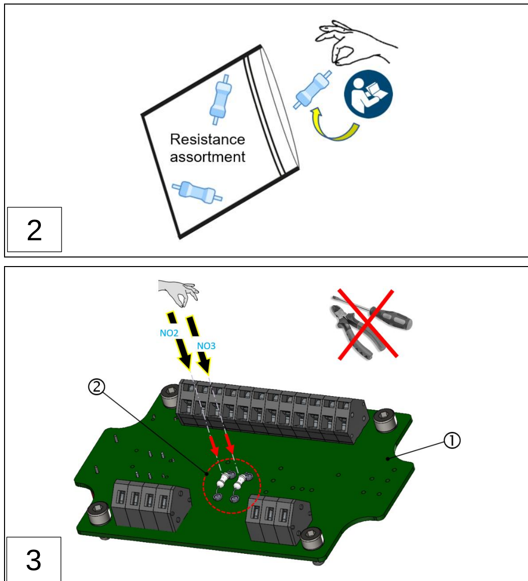
Abb.: 45 : Klemmenkasten VN200: Drahtbruchwiderstände einsetzen (Montageschritte 1-3)
