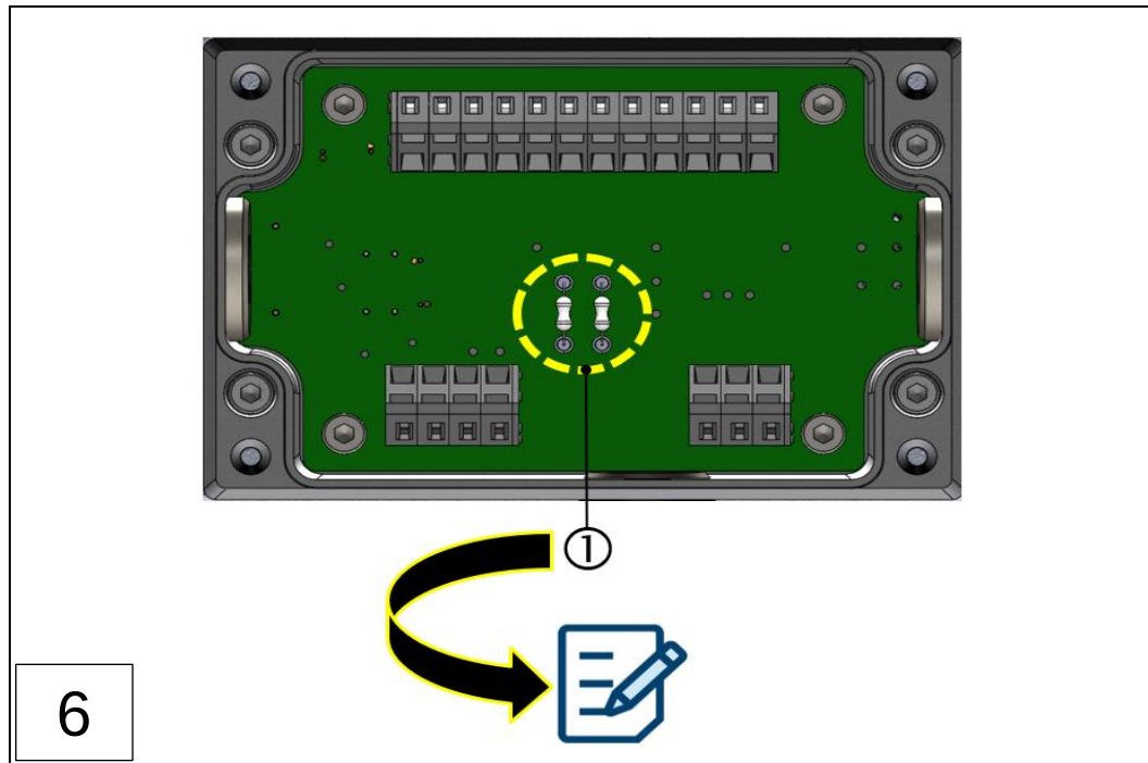
1: Drahtbruchwiderstände
