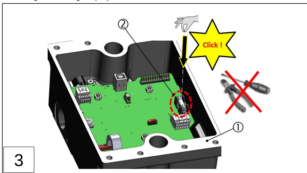
Abb.: 85 :Sicherung am Messaufsatz austauschen, VN2020 (Schritte 1-3)
