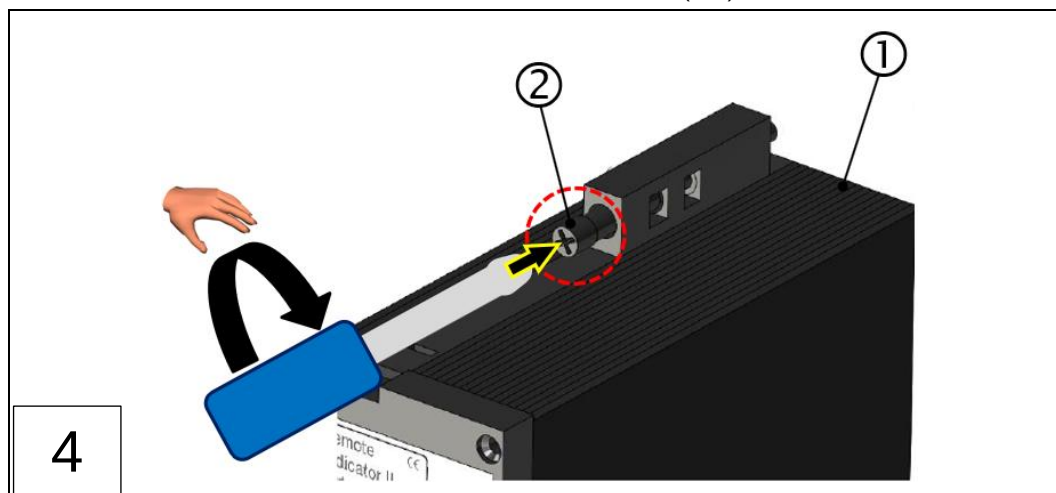
Abb.: 40 : Montage Remote Indicator II (Montageschritte 1-4)
