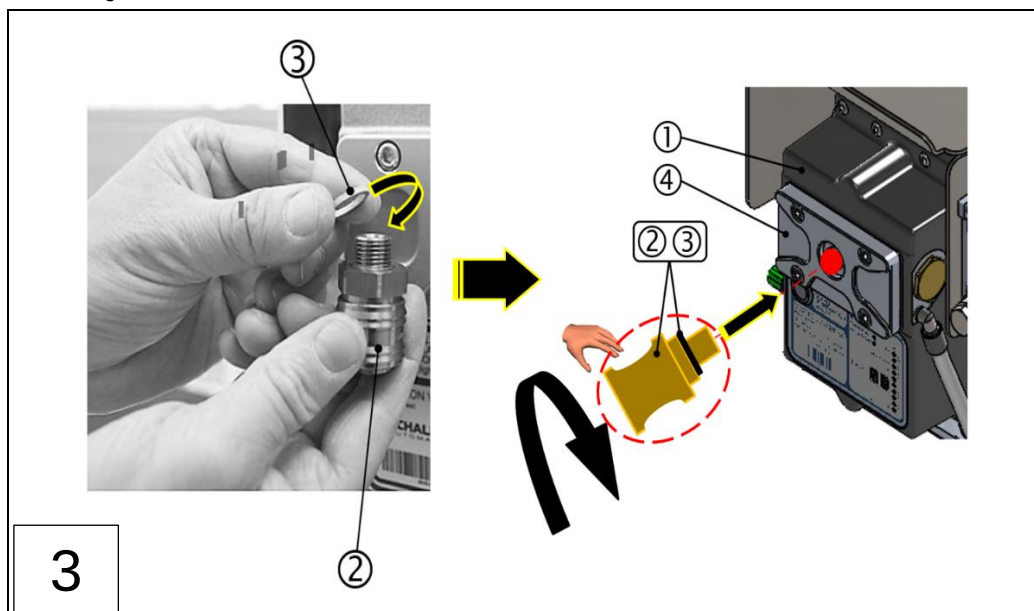
1: Messaufsatz 3: Dichtring
