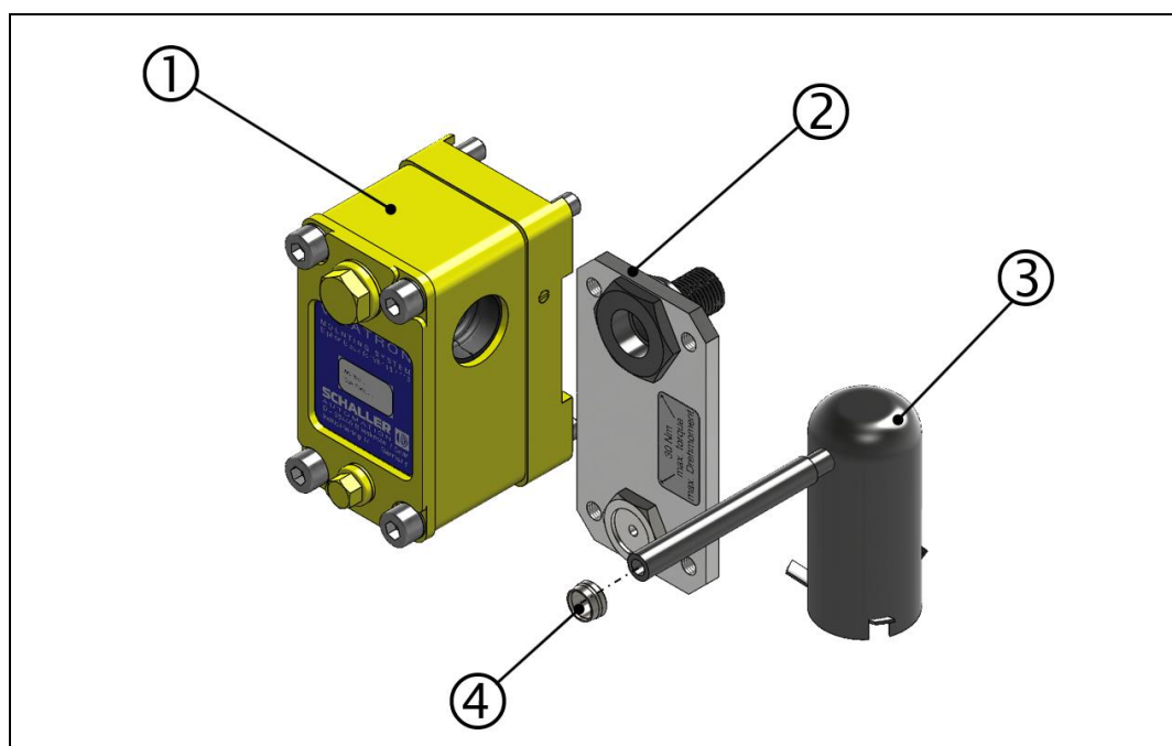
Abb.: 30 :Siphonblock- Baugruppe
