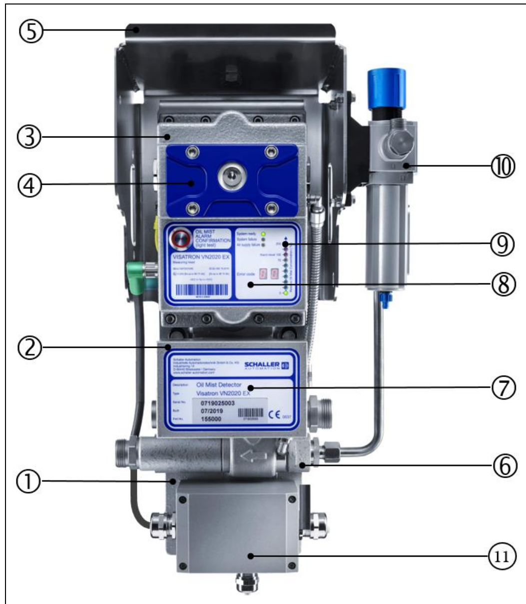
Abb.: 13 :Komponentenübersicht, Ölnebeldetektor VISATRON® VN2020 EX
