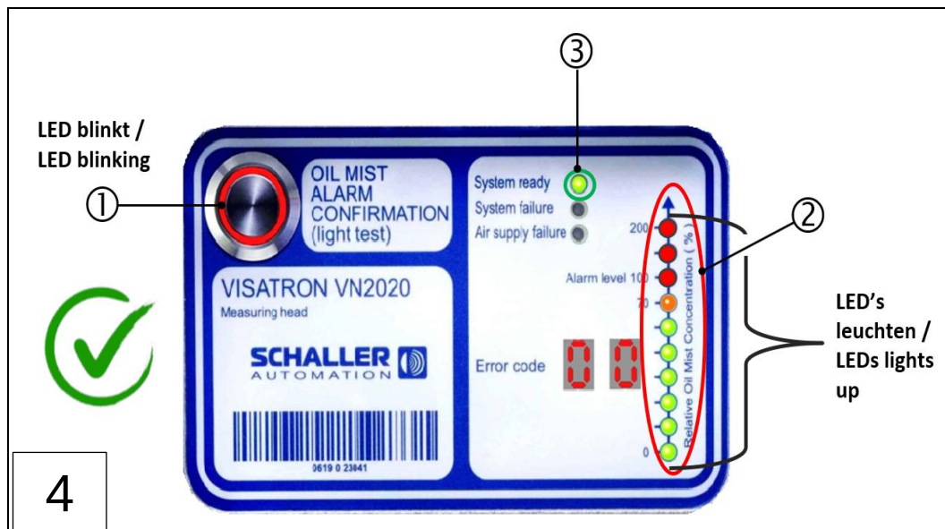
Abb.: 80 : Funktionstest mit Testnebel (Schritte 1-4)
