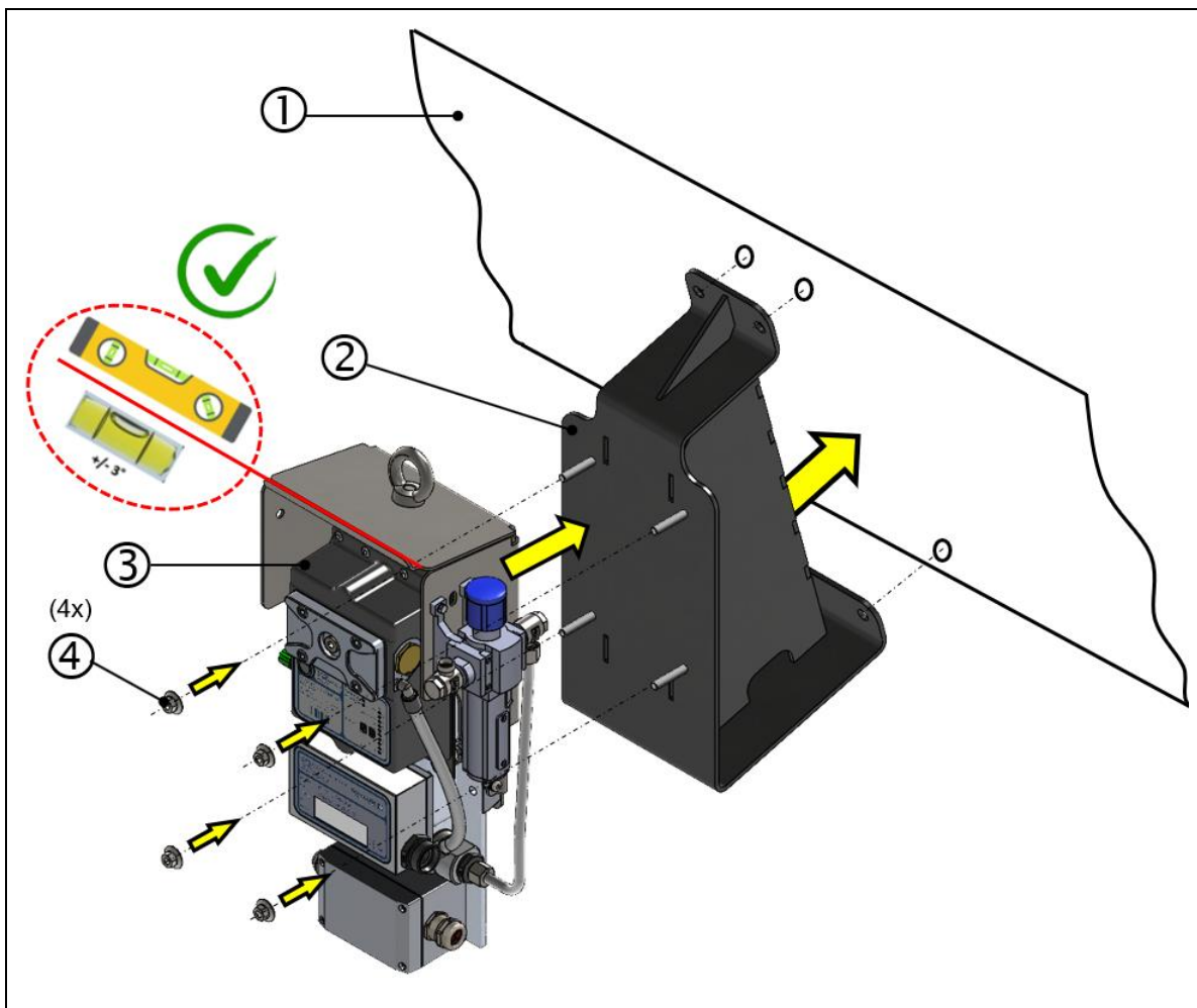
Abb.: 24 :Montagevorgang, VN2020 mit Konsole und Schutzhaube
