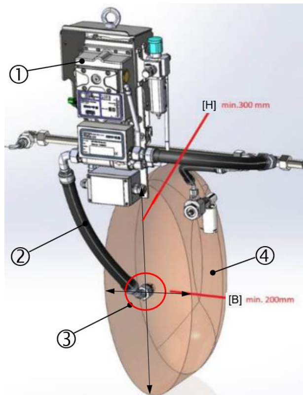
Abb.: 35 : Position der Rückführungsleitung, VN2020
