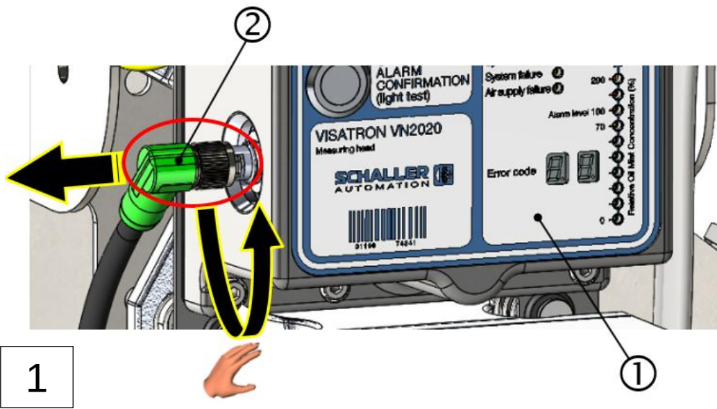
1: Messaufsatz, VN2020
