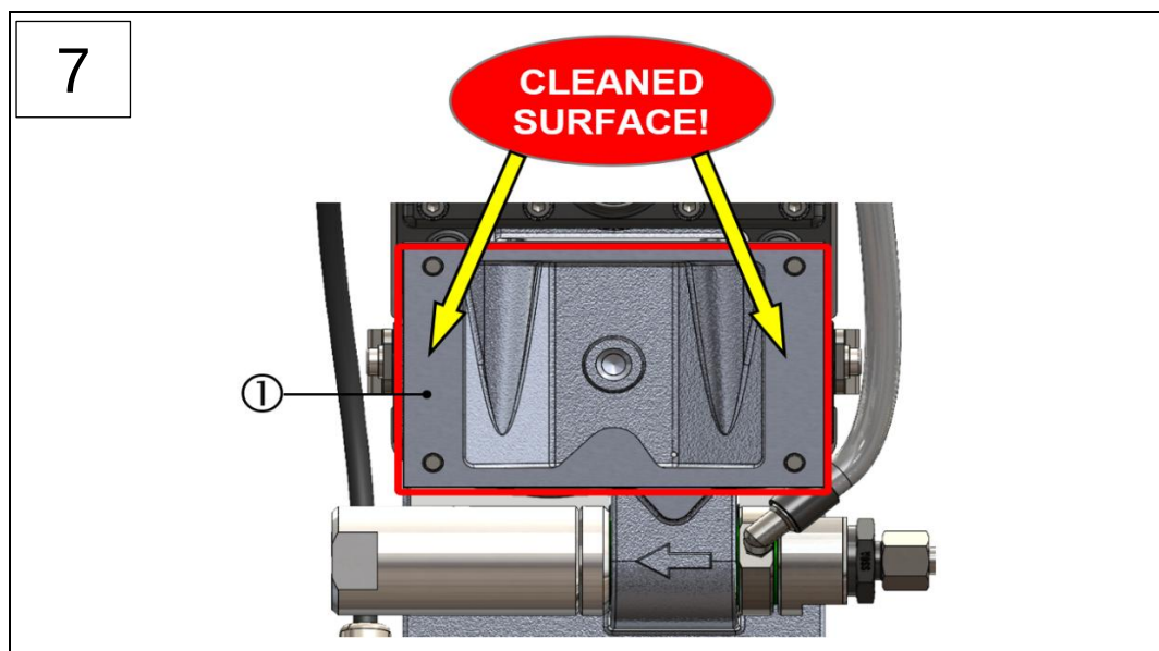
1: Dichtungsfläche "Anschlusskasten"
