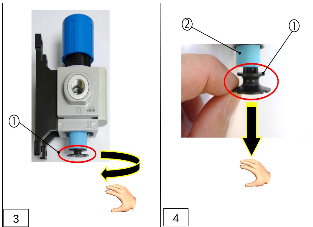
1: Kunststoff- Drehscheibe
