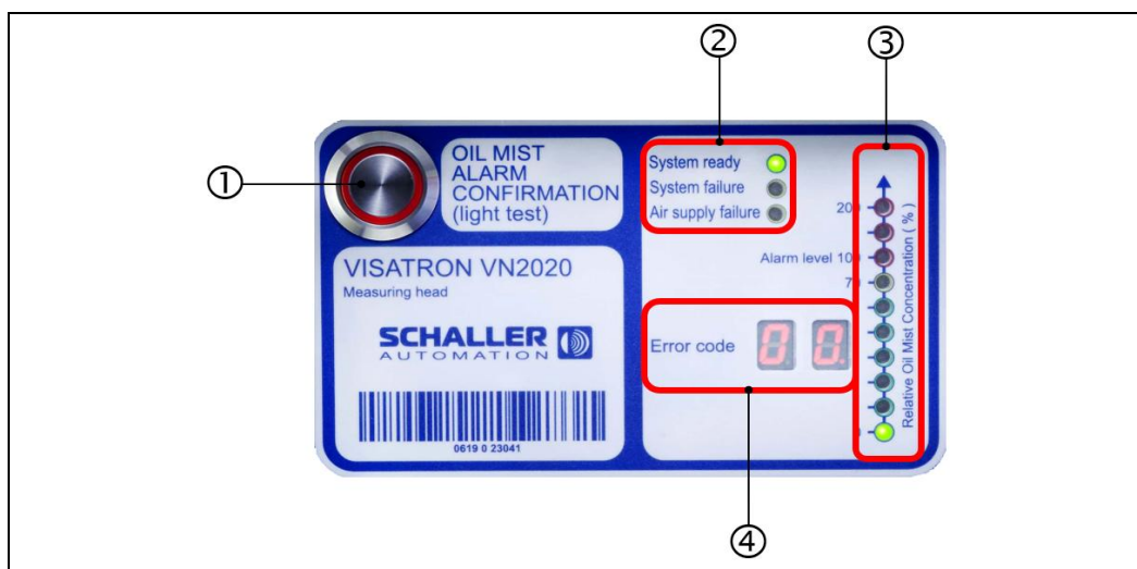
Abb.: 22 :Bedien- und Anzeigeelement, VN2020
