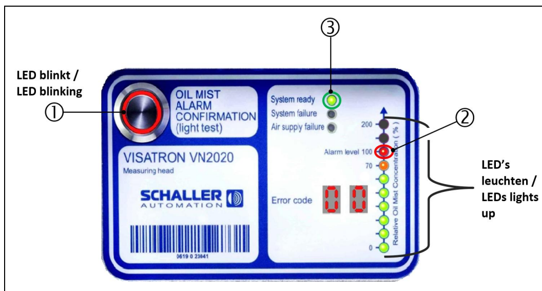
Abb.: 72 :Messaufsatz VN2020: Status- Anzeige „Alarm“ bei 100% ÖNK
