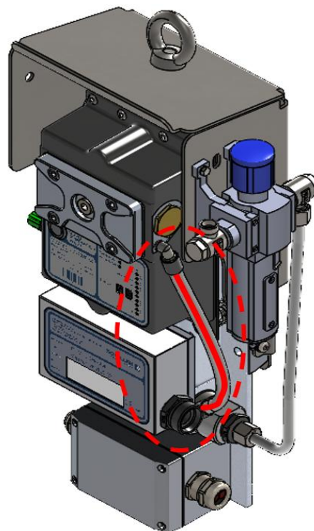
Abb.: 92 :Verbindungsschlauch, Ölnebeldetektor VN2020
