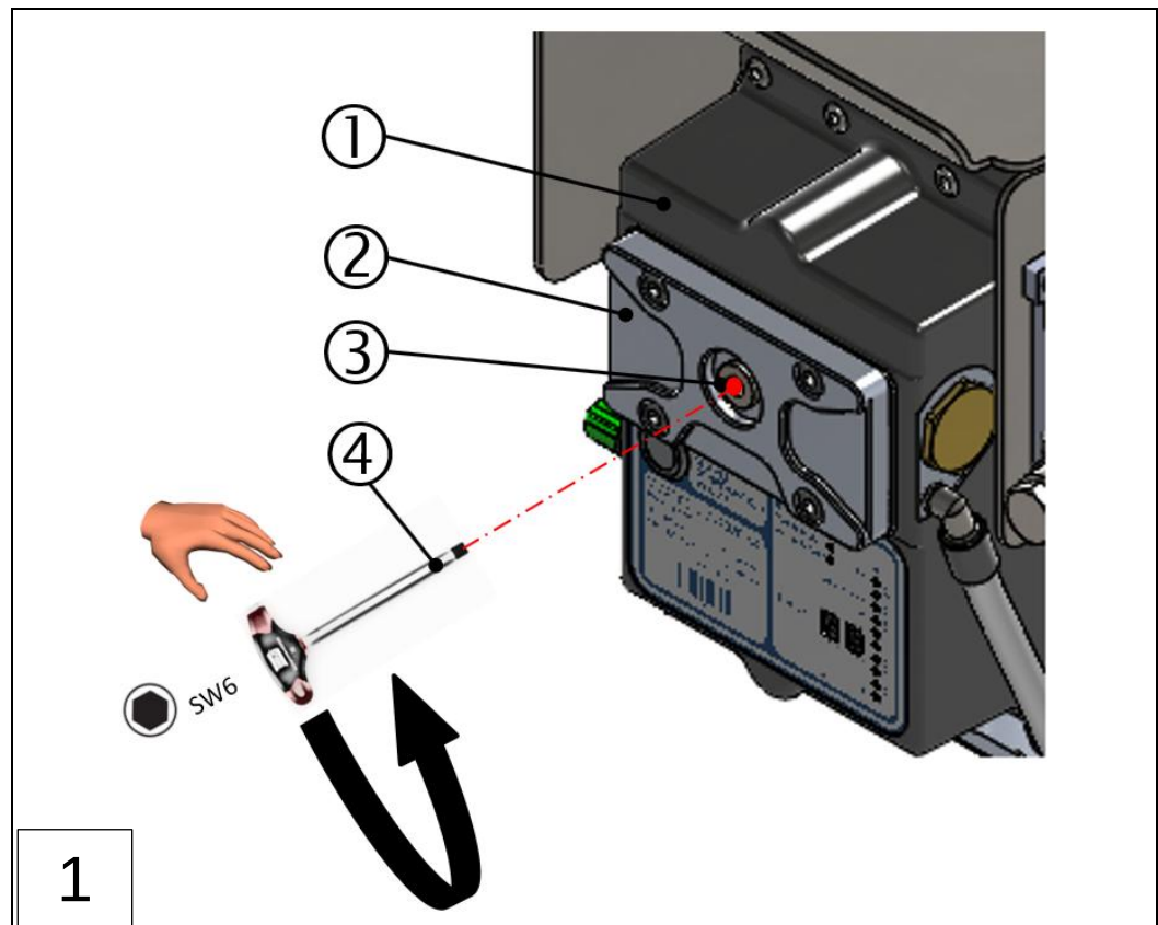
1: Messaufsatz 3: Verschlusschraube
