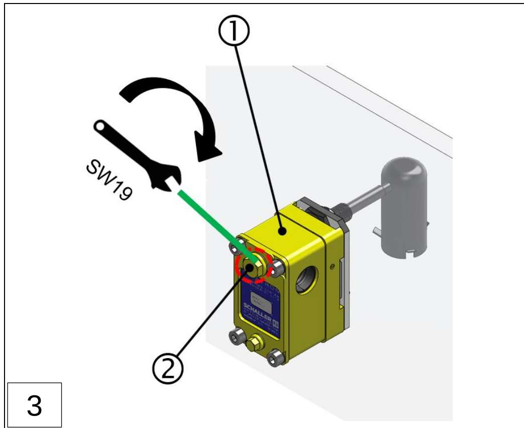
Abb.: 64 :Werktest mit Rauchgenerator (Schritte 1-3)
