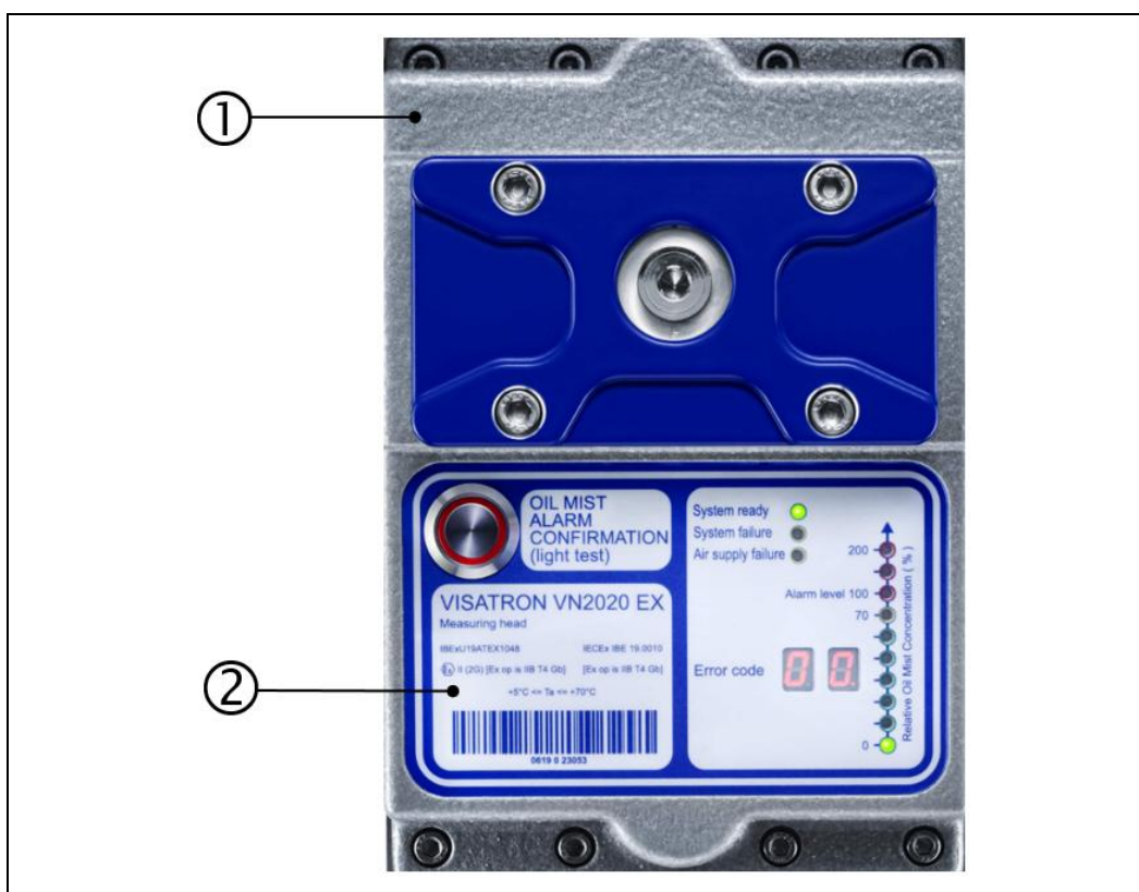
Abb.: 3 : Typenschild, Messaufsatz VISATRON® VN2020 EX
