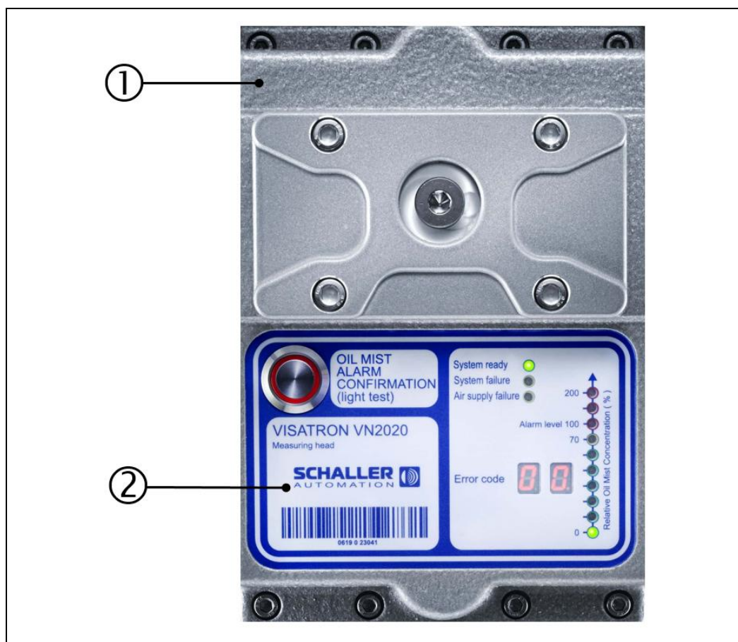
Abb.: 1 : Typenschild, Messaufsatz VISATRON® VN2020
