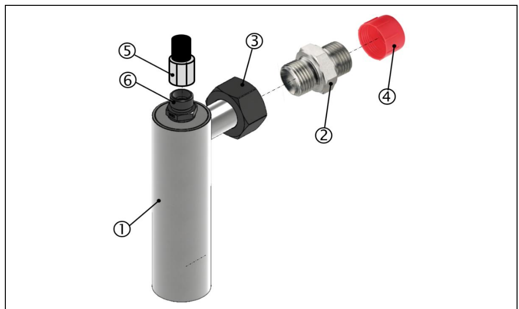
Fig.: 21 : Pipe siphon assembly
