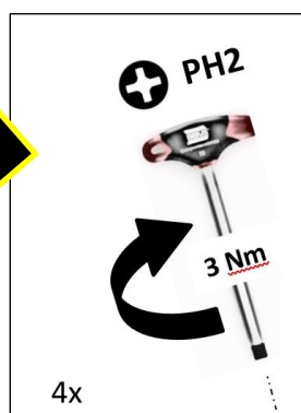
图：80：锁闭 VN301 plus 中央单元（步骤 1-4）
