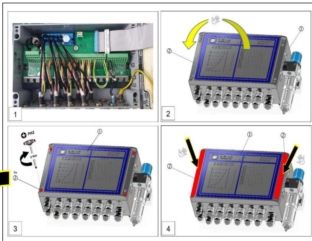
图：80：锁闭 VN301 plus 中央单元（步骤 1-4）
