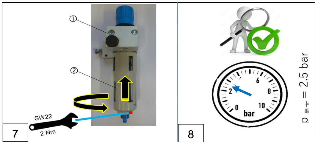
图: 96: 更换空气滤清器滤芯, 压力控制器单元 (步骤 1-8)
