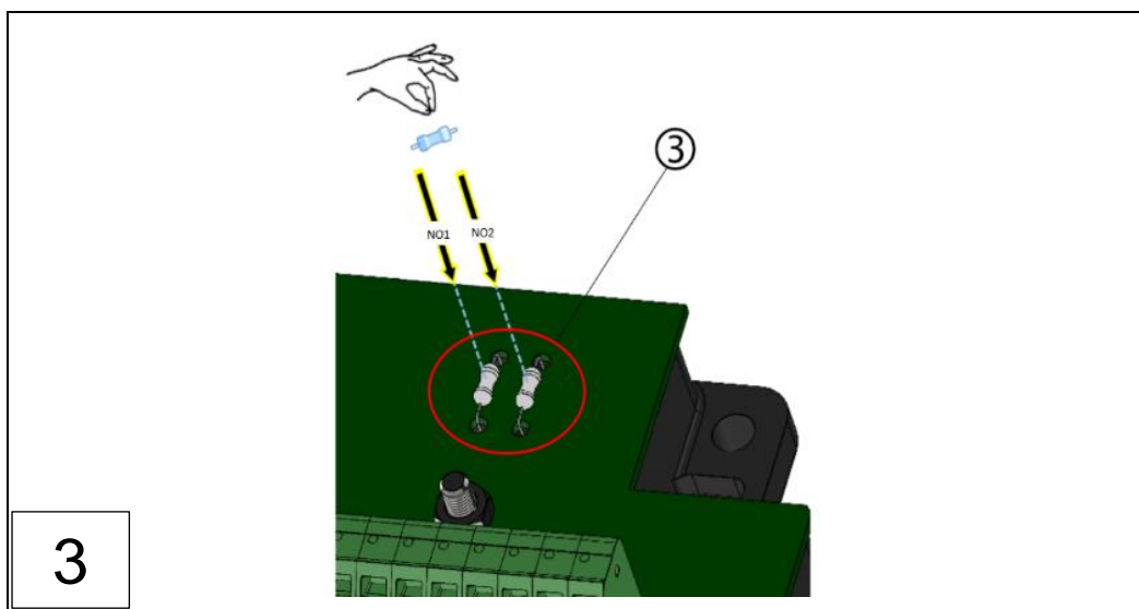
图 : 57 : VN301 plus 中央单元 : 装入断路电阻 (装配步骤 1-3)
