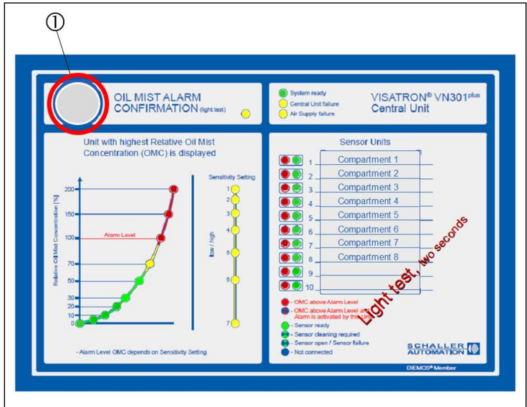
图：83：VN301 plus 中央单元：LED 检查（指示灯测试）
