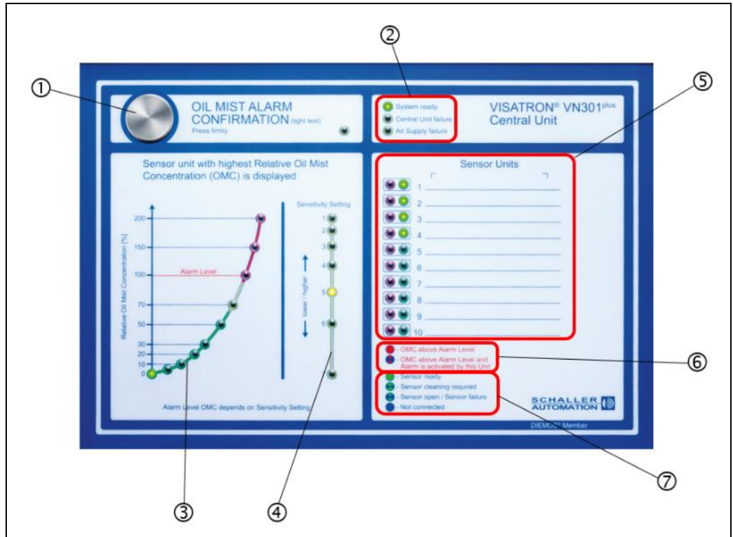
图：23：操作与显示元件，VN301plus 中央单元
