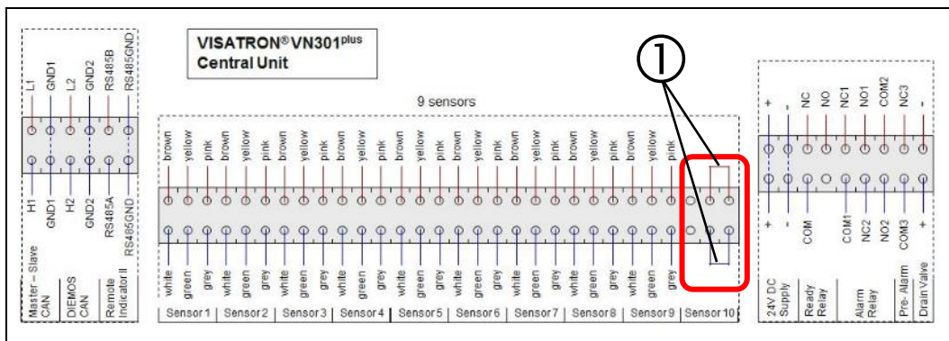
图：63：VN301 plus 中央单元：接线桥的配置，9 个传感器
