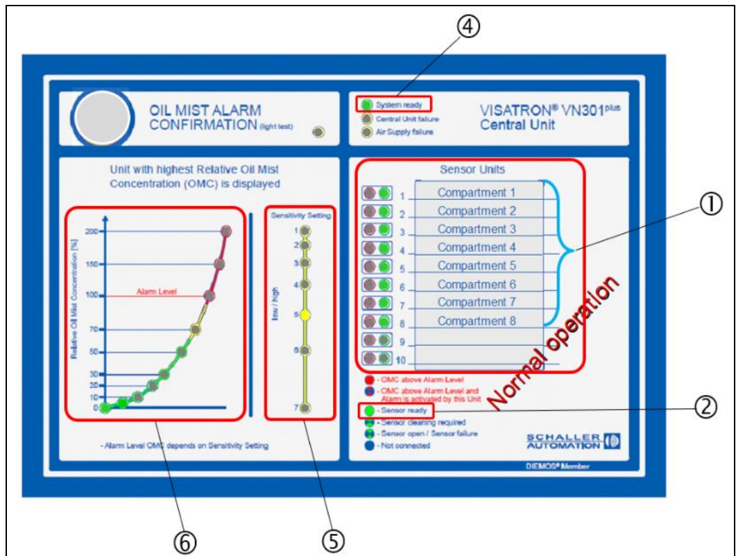
图：81：VN301plus 中央单元：正常运行时的显示（无油雾报警，无故障）
