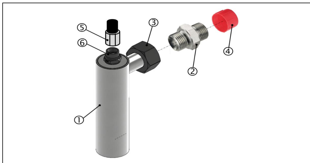
Fig.: 32 : Pipe siphon assembly
